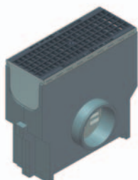
odtoková vpust s litinovým pororoštem, tř. D 400, s aretací
